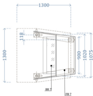
VUE DESSUS
